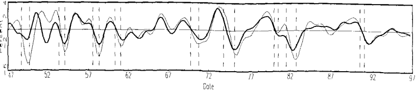
Fig. 3.9. Consumption (total).
