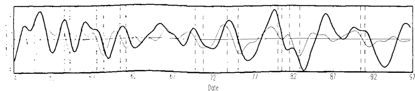
Fig. 3.60. Consumer credit.
